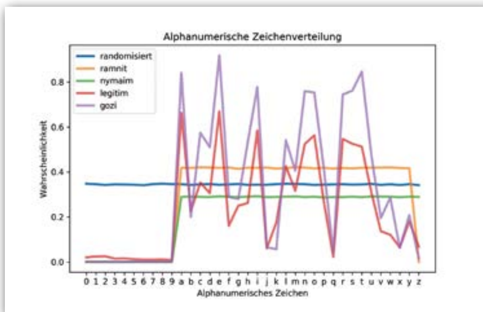
Verteilung alphanumerischer Zeichen von legitimen Domännennamen (ALEXA & MAJESTIC), randomisierten DGAs (ramnit, nymaim), wort-basiertem DGA (gozi) und zufällige alphanumerischen Zeichen.
