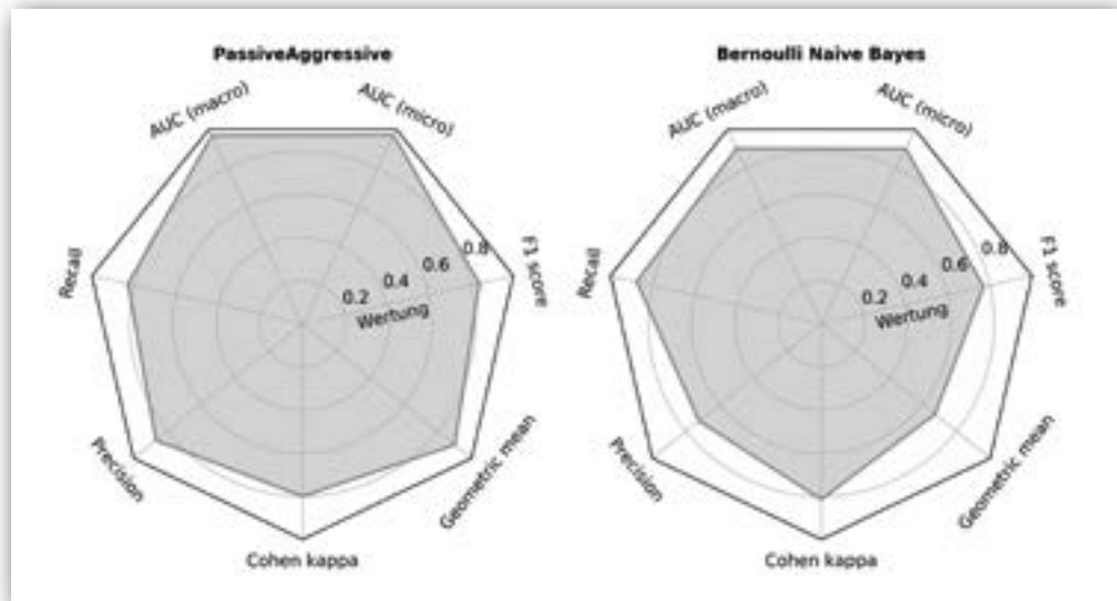
Vergleich verschiedener Metriken für zwei Klassifikatoren. Werte näher an 1.0 sind besser.
